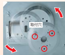
丸刃偏芯軌道 丸刃に取付穴が3カ所あり、取付位置が変更できます。
